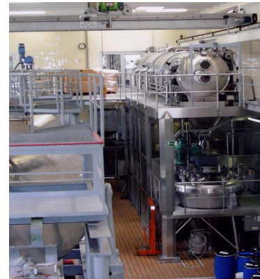
(殺菌・有害物質除去装置)
